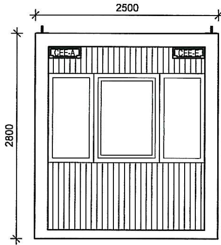
Aussenansicht SBL A WE4 Container Flur WE mit ZK-Tür u. Fenster
