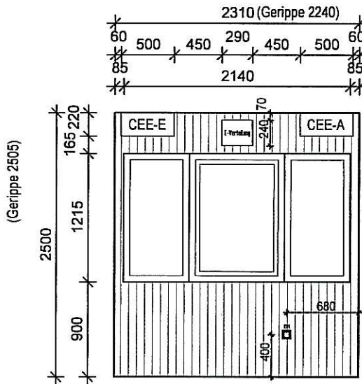
Innenansicht SBL A WE4 Container Flur WE mit ZK-Tür u. Fenster
