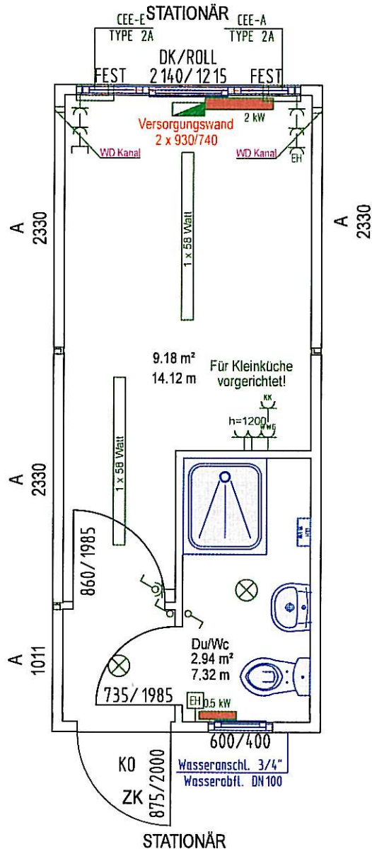
TYP SBL A6-1.7 Container Leer mit WC und Dusche
